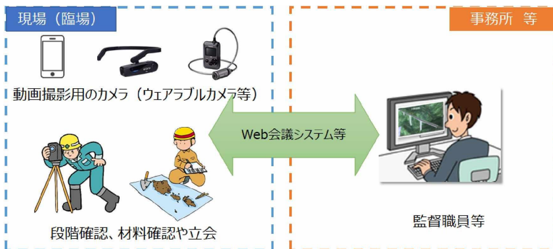
図 2-1 機器構成 (例)
